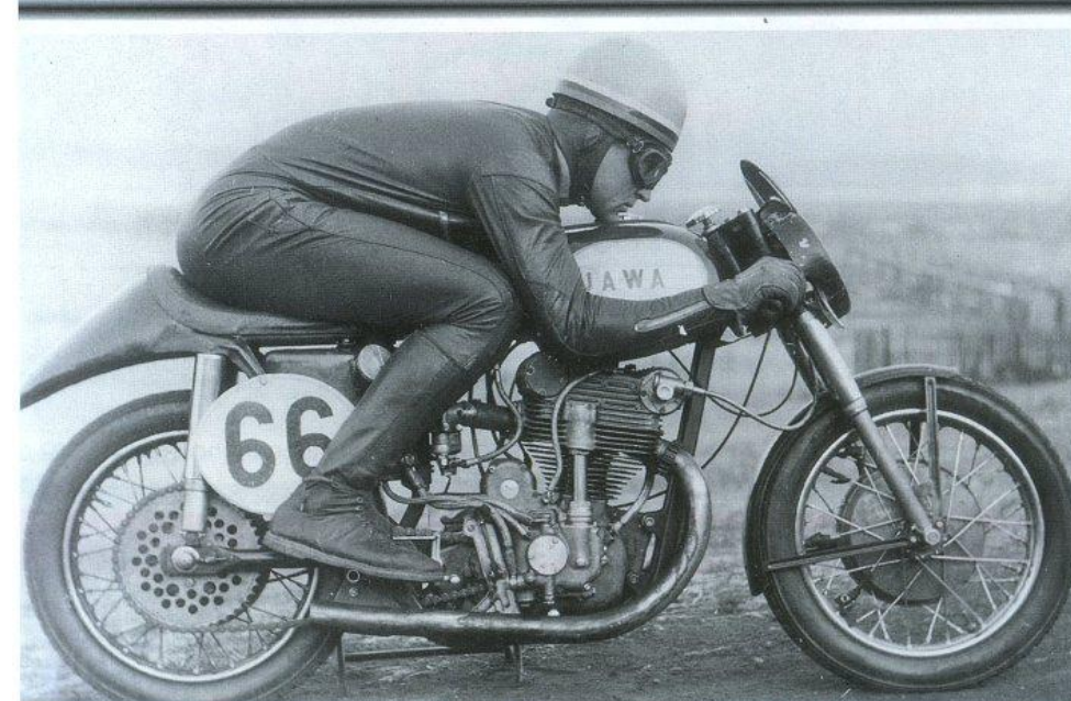
F. Šťastný Jawa 250 2x OHC příprava na den rekordů 1953.
