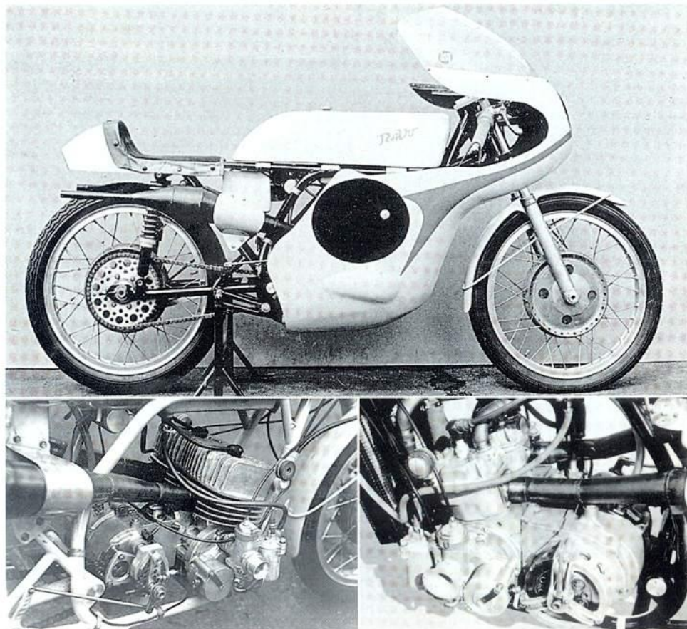
RAVO 4, 1968 - 1975, vlevo vzduchem a vpravo vodou chlazený motor 125 ccm
